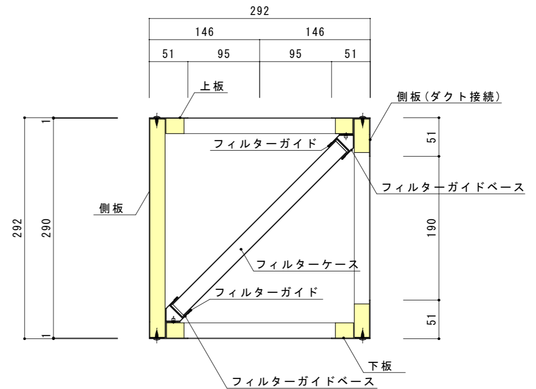
断熱フィルターボックス 断面図
