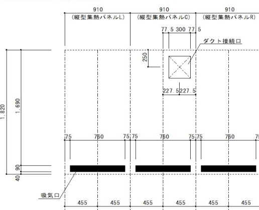
縦設置型集熱パネルの場合
