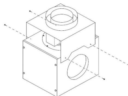
電動ダンパー固定板の取付
