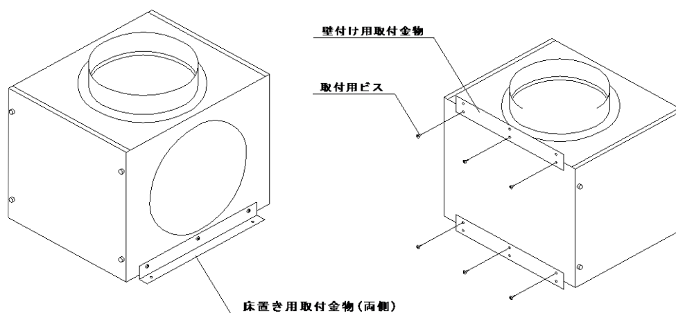
床置き用取付金物
