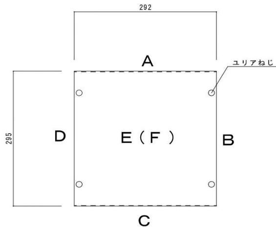
側面(フィルタ ー蓋)
