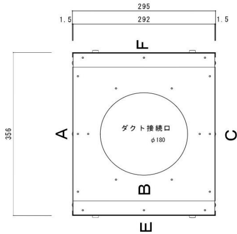
側面(ダクト 接続側)
