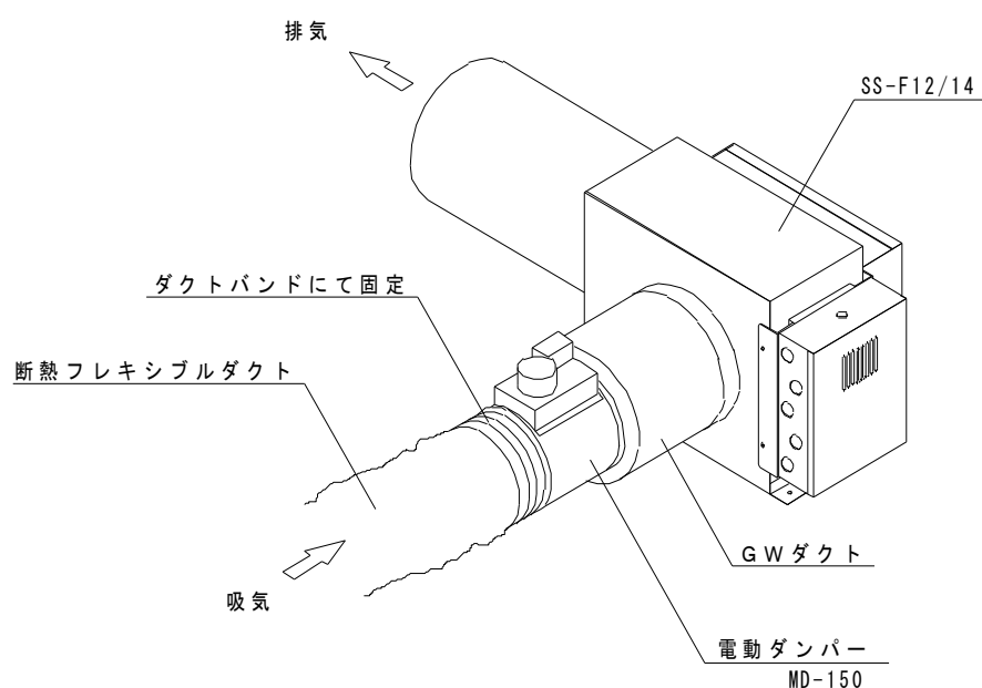
電動ダンパー使用例
