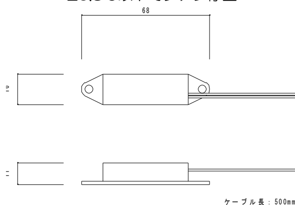
温度スイッチ 外形寸法
