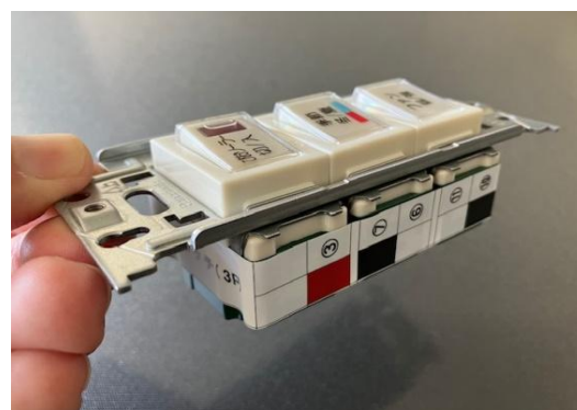
スイッチ側面の配線番号指示
