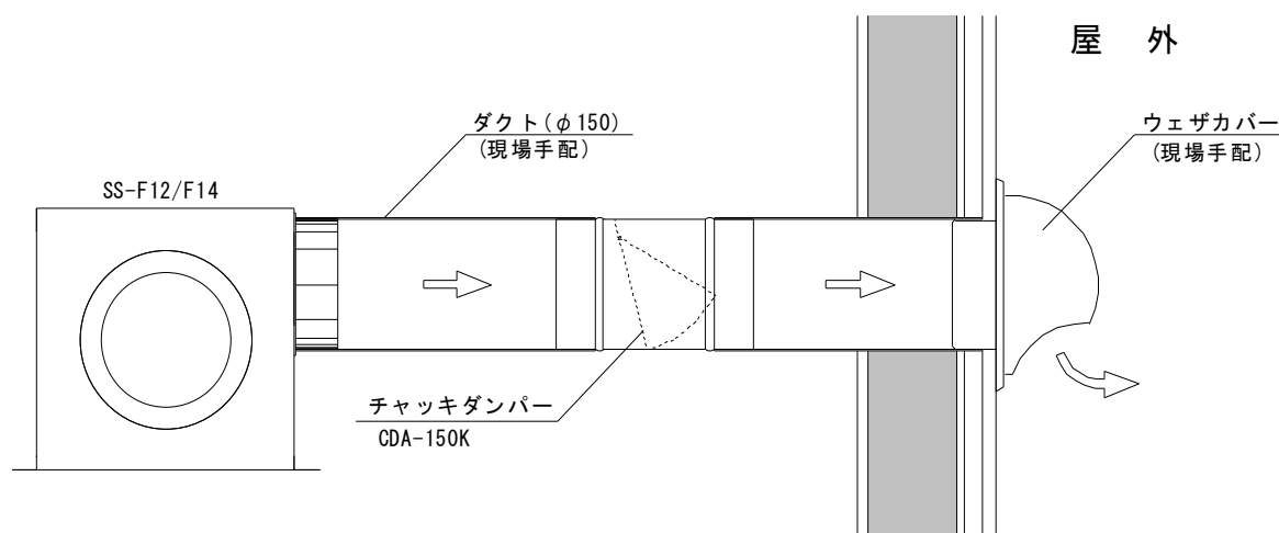
チェックダンパー使用例
