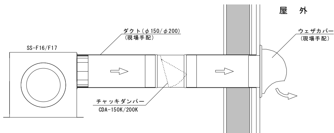
チャッキダンパー使用例
