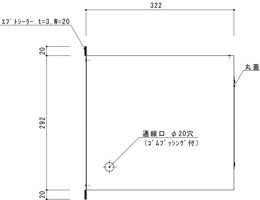
側面
