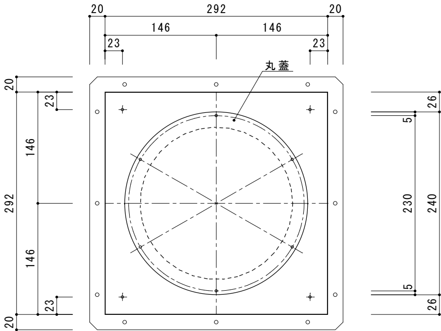
正面
