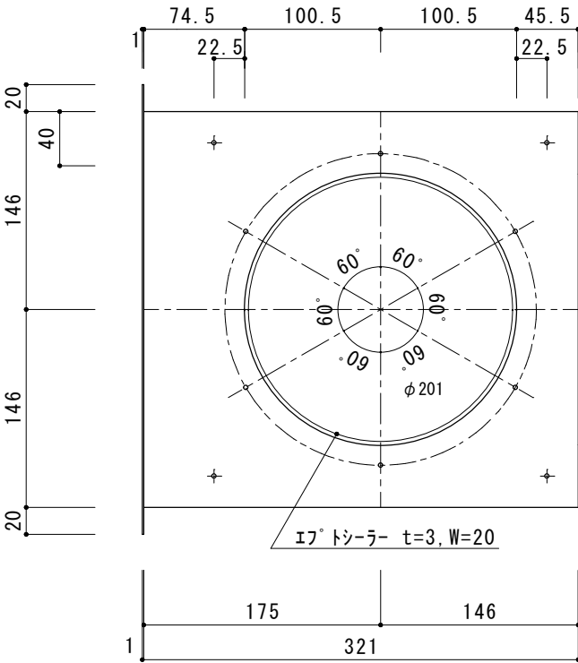
底面
