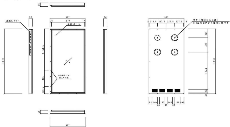
縦型集熱パネル RD仕様
