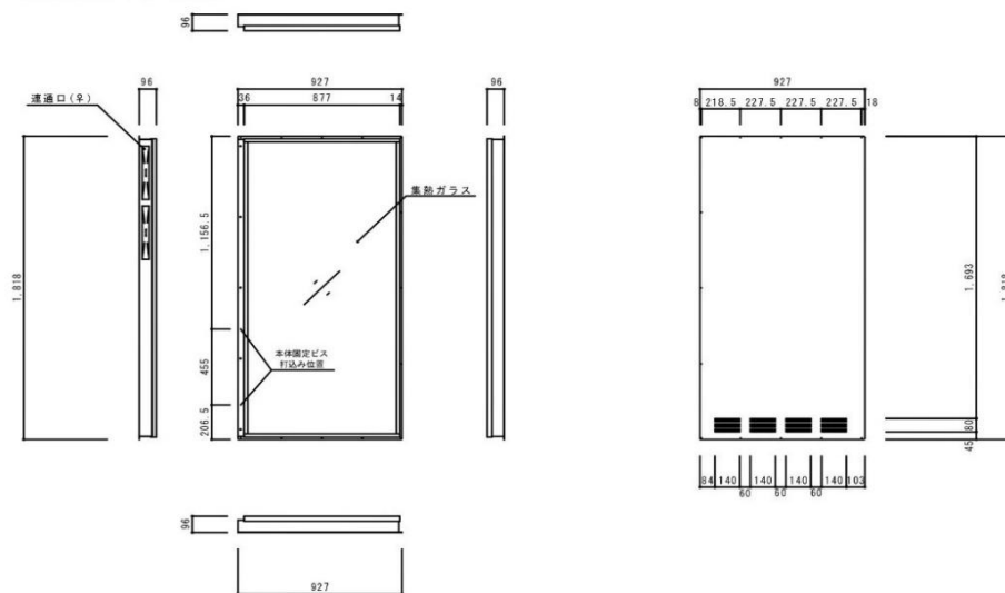
縦型集熱パネル R仕様
