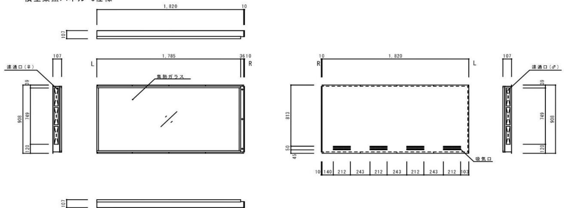
横型集熱パネル C仕様
