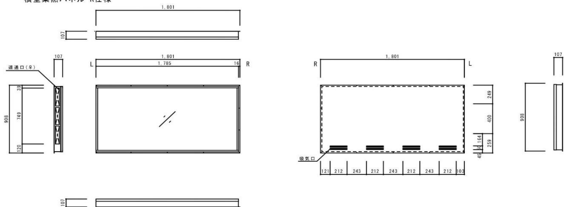
横型集熱パネル R仕様
