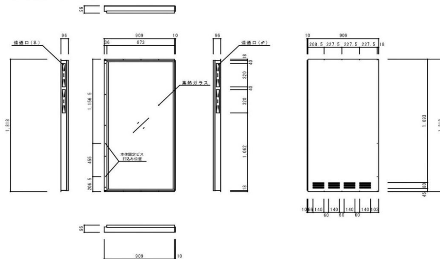
縦型集熱パネル O仕様
