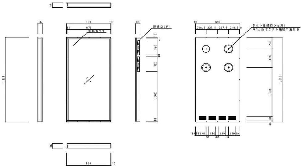
縦型集熱パネル LD仕様
