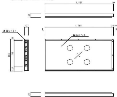
横型集熱パネル RD仕様
