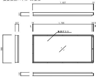
横型集熱パネル CD仕様
