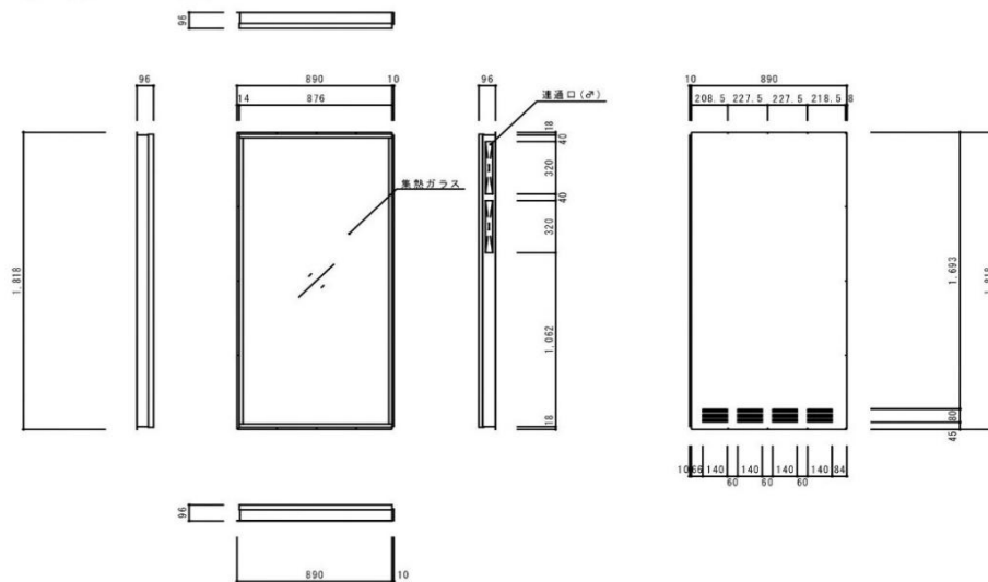
縦型集熱パネル L仕様
