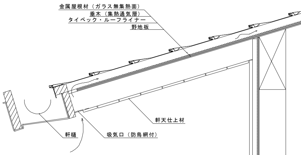
軒先・吸気口廻り納まり図
