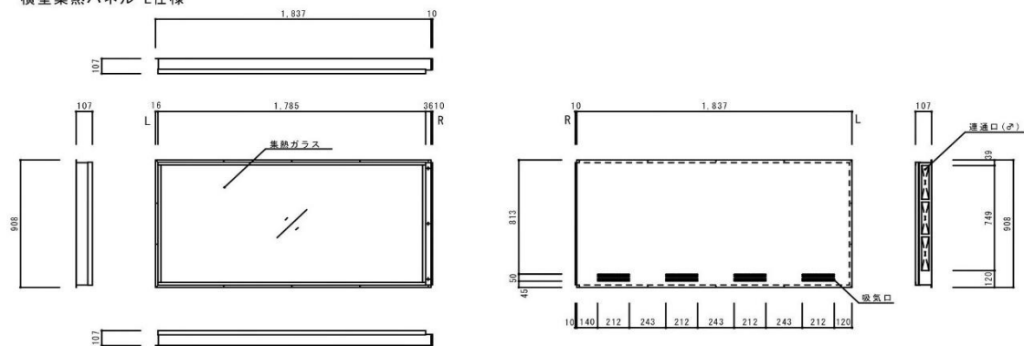
横型集熱パネル L仕様
