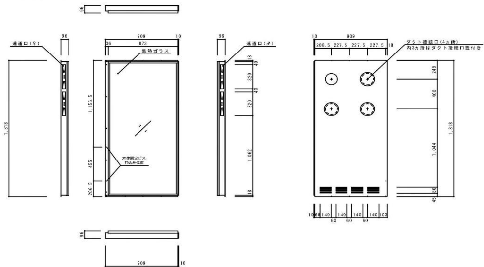
縦型集熱パネル CD仕様
